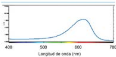
Espectro visual
